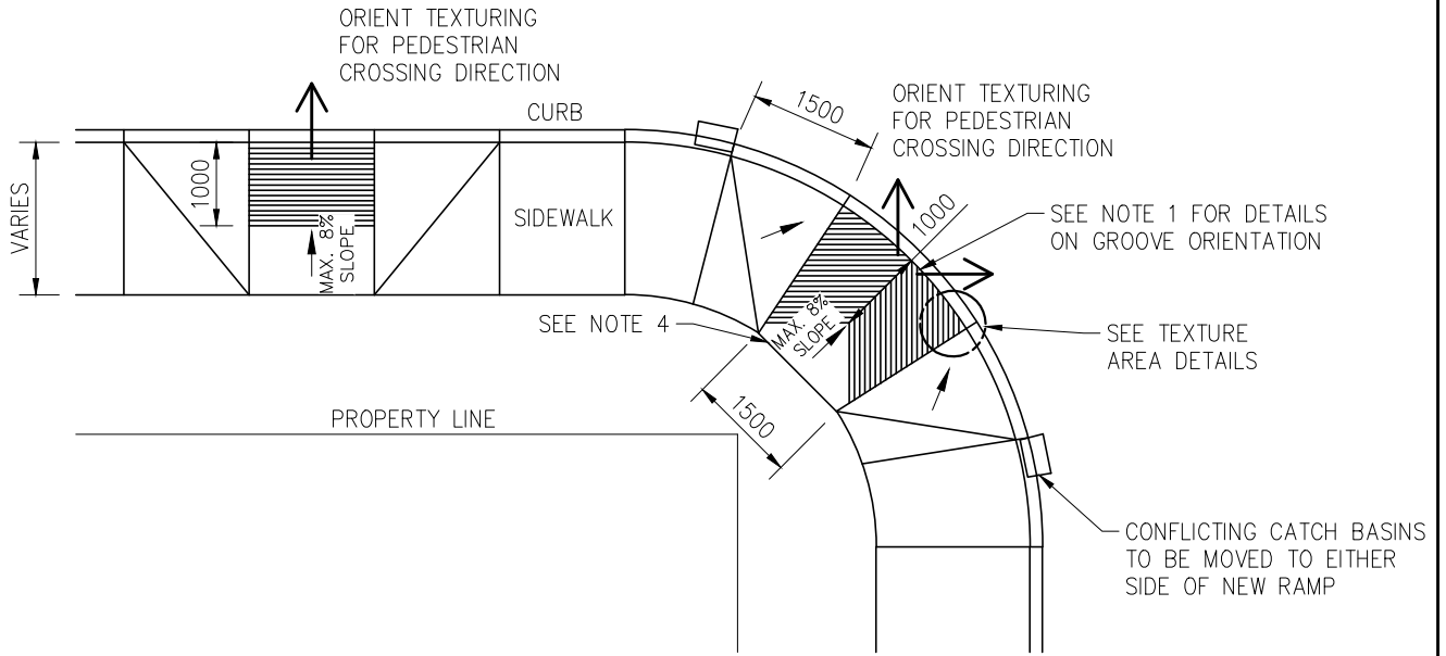
PEDESTRIAN RAMP SCALE N.T.S.
