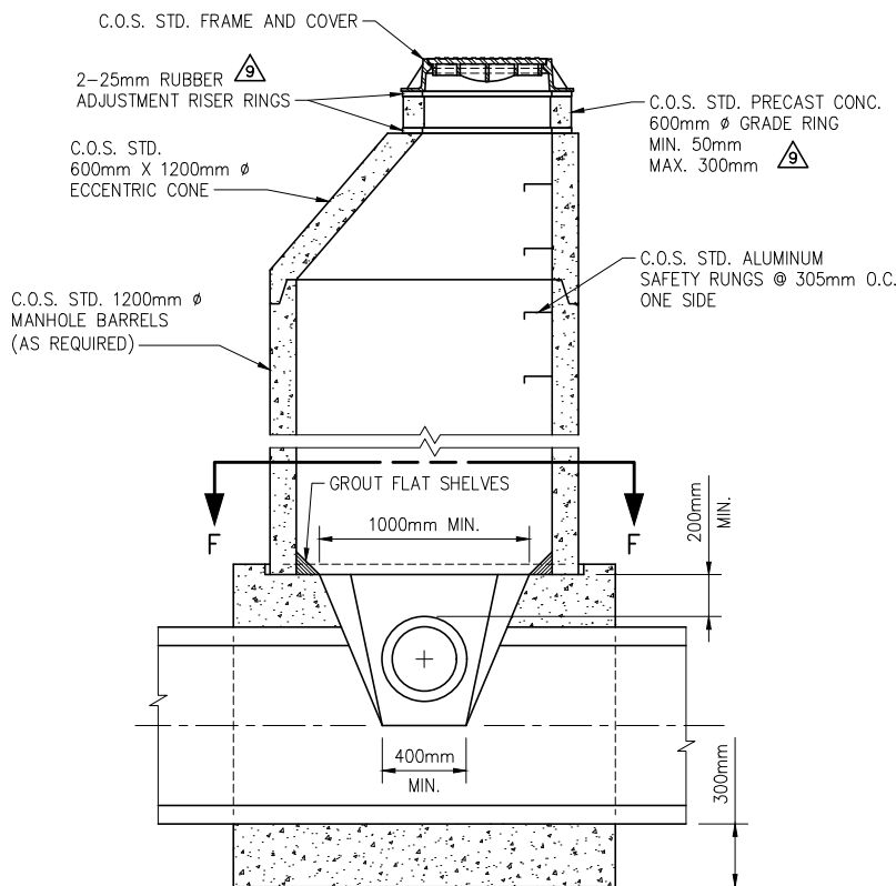
SECTION D-D
