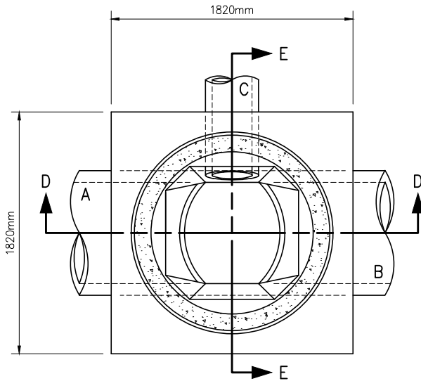
SECTION D-D
